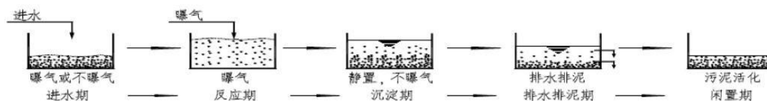
图 3-4 SBR 内部处理流程
