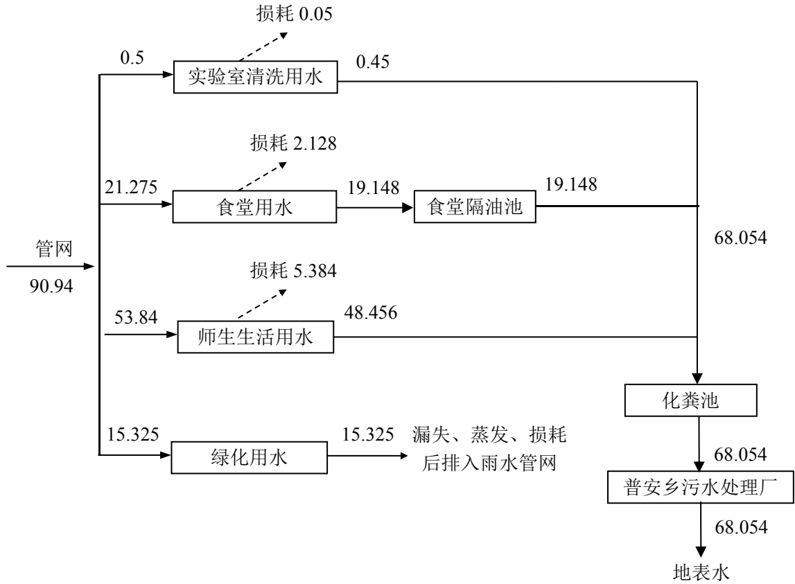
图 3-1 项目水平衡分析图 单位：m 3 /d
