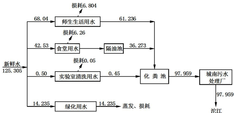
图 3-1 项目水平衡分析图 单位：m 3 /d
