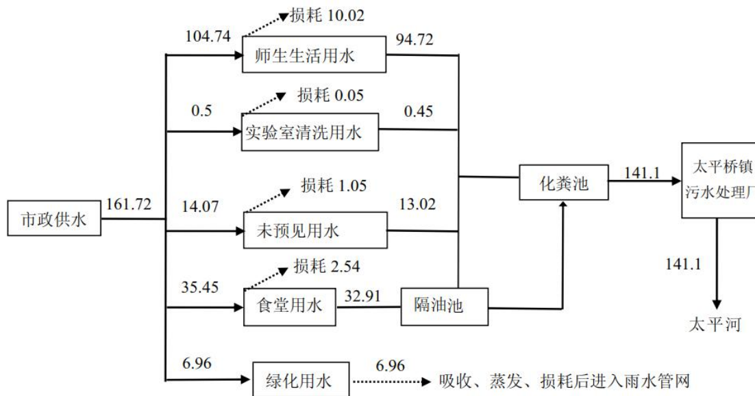
图 3-1 项目水平衡分析图 单位: m 3 /d
